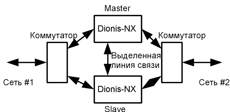
Рис. 57.1: Отказоустойчивый аппаратный кластер
