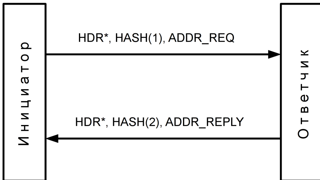
Рис. 55.4: Фаза ModeConfig
