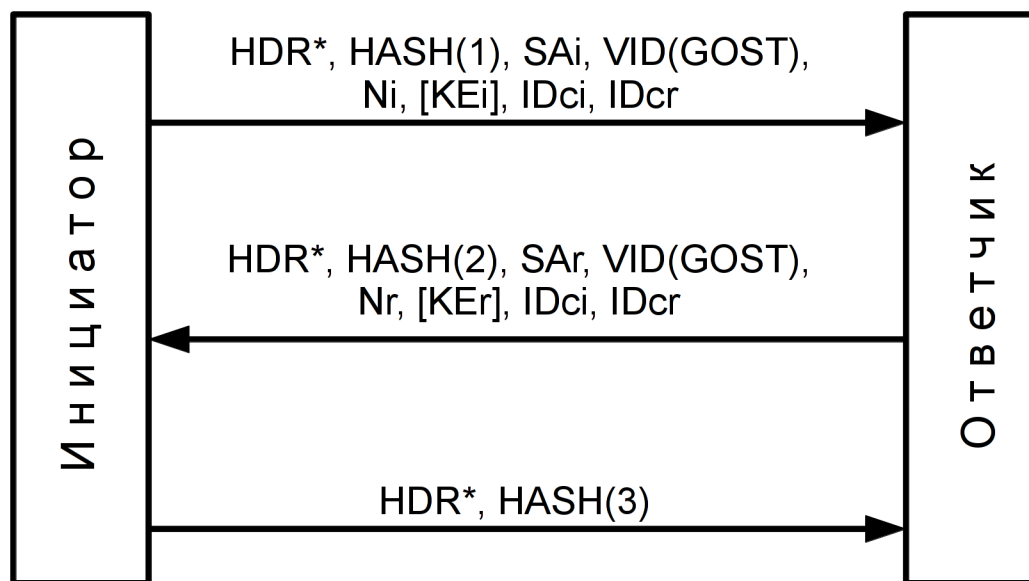
Рис. 55.3: Фаза 2
