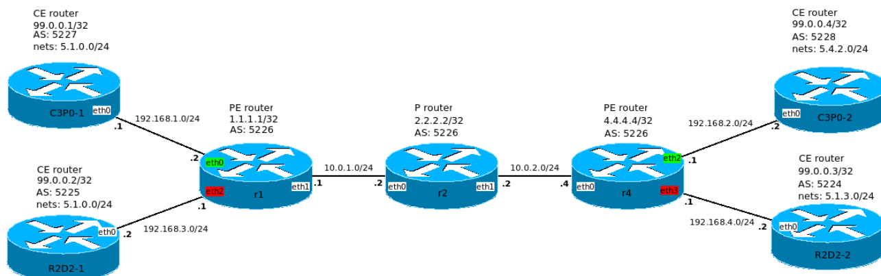
Рис. 54.2: Схема 2: MPLS-L3VPN
