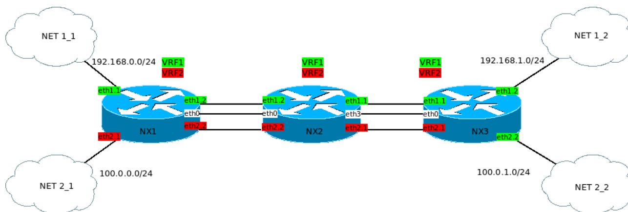
Рис. 54.1: Схема 1: vrf-lite + OSPF
